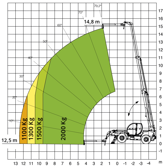
Diagramma portate Jib 2.000 kg
