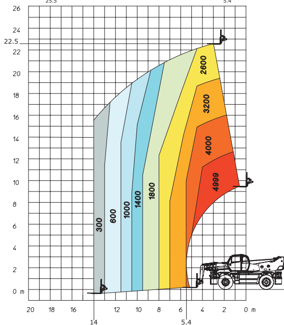
Frontale su pneumatici con forche
