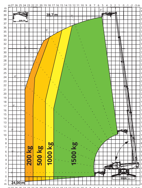
JIB CON ARGANO 1.500 kg
