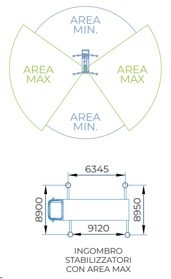
MAN TGM 18.290 - 4X2 BB CH - PASSO 3875
